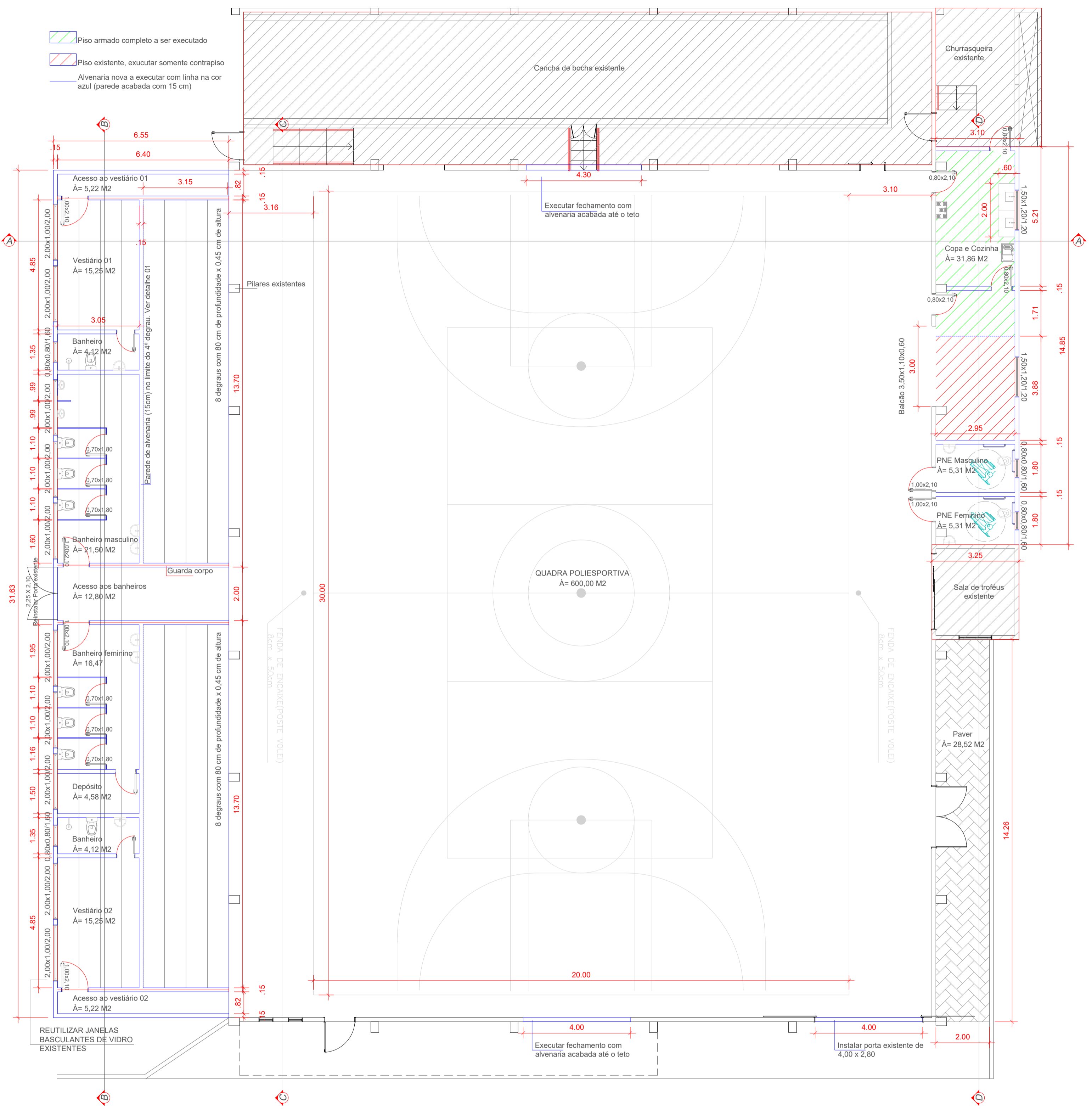
02 PLANTA BAIXA ESC.: 1:100
